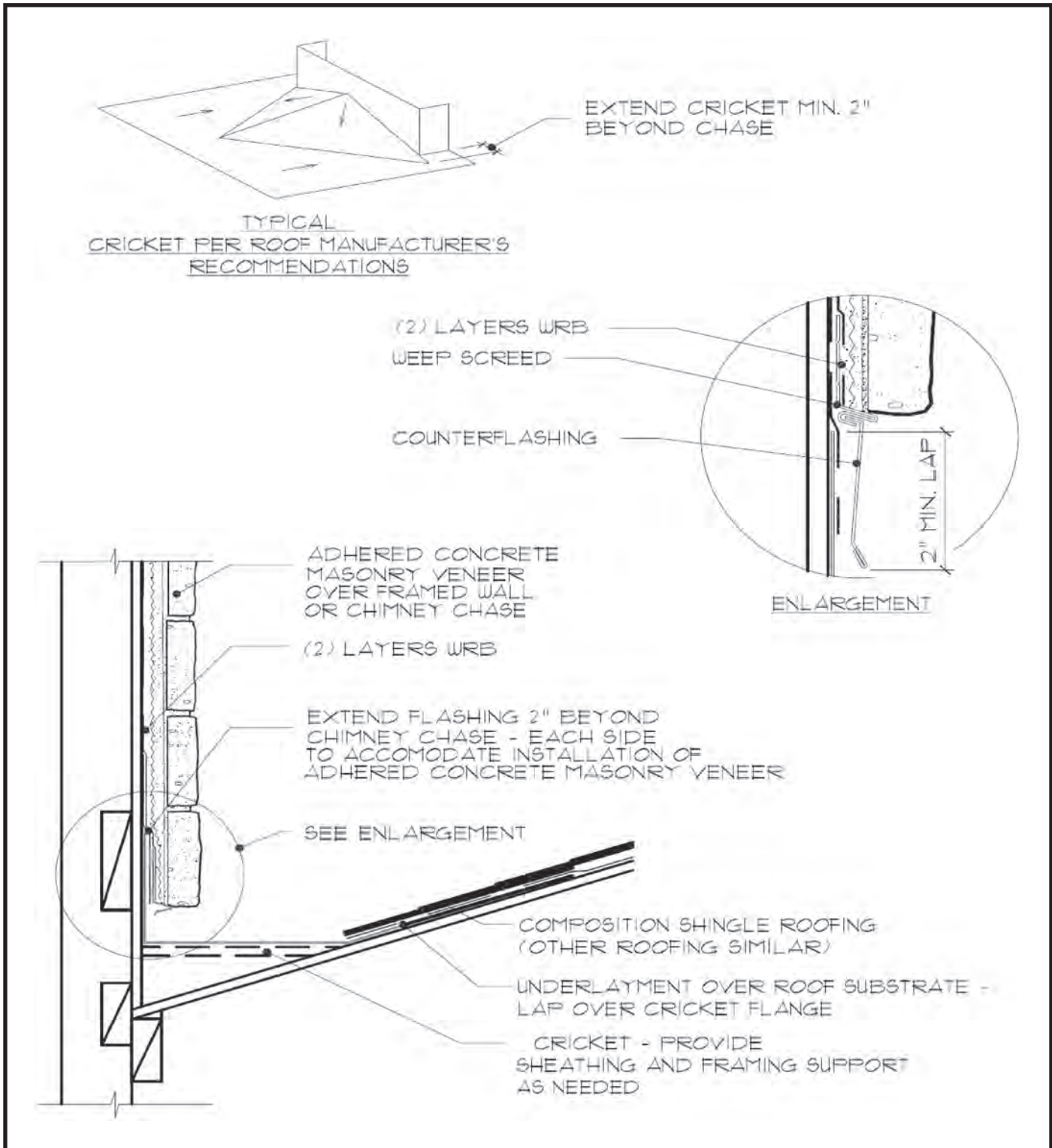
Fig. 23. Cricket
