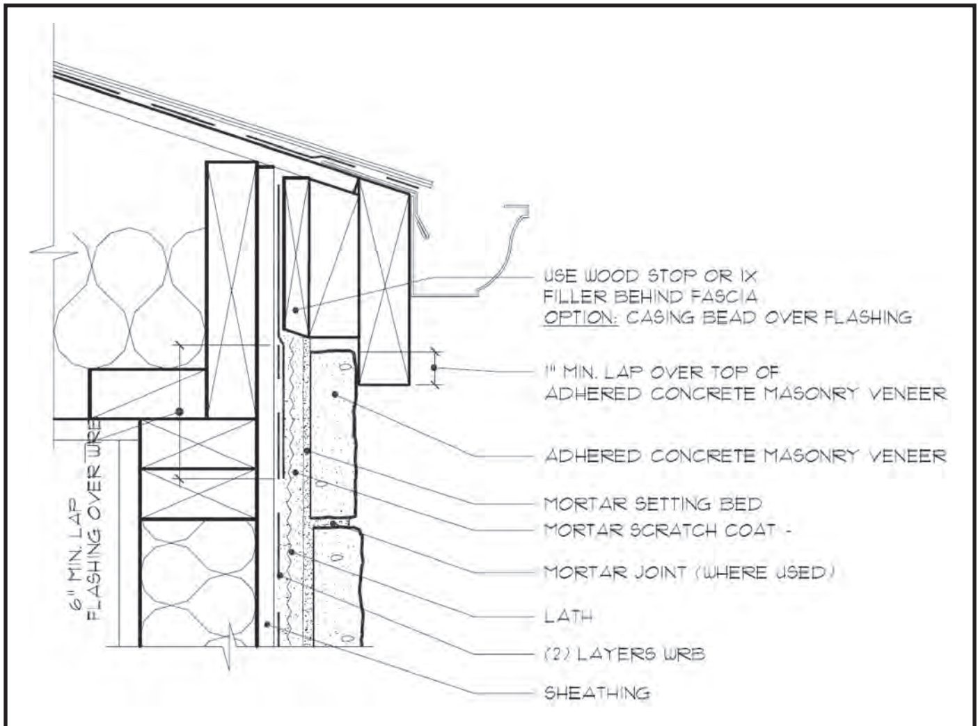
Fig. 12. Open Eave - Flush
