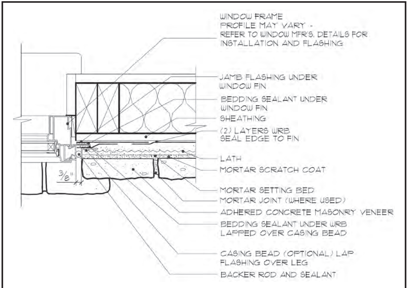
Fig. 20. Window Jamb
