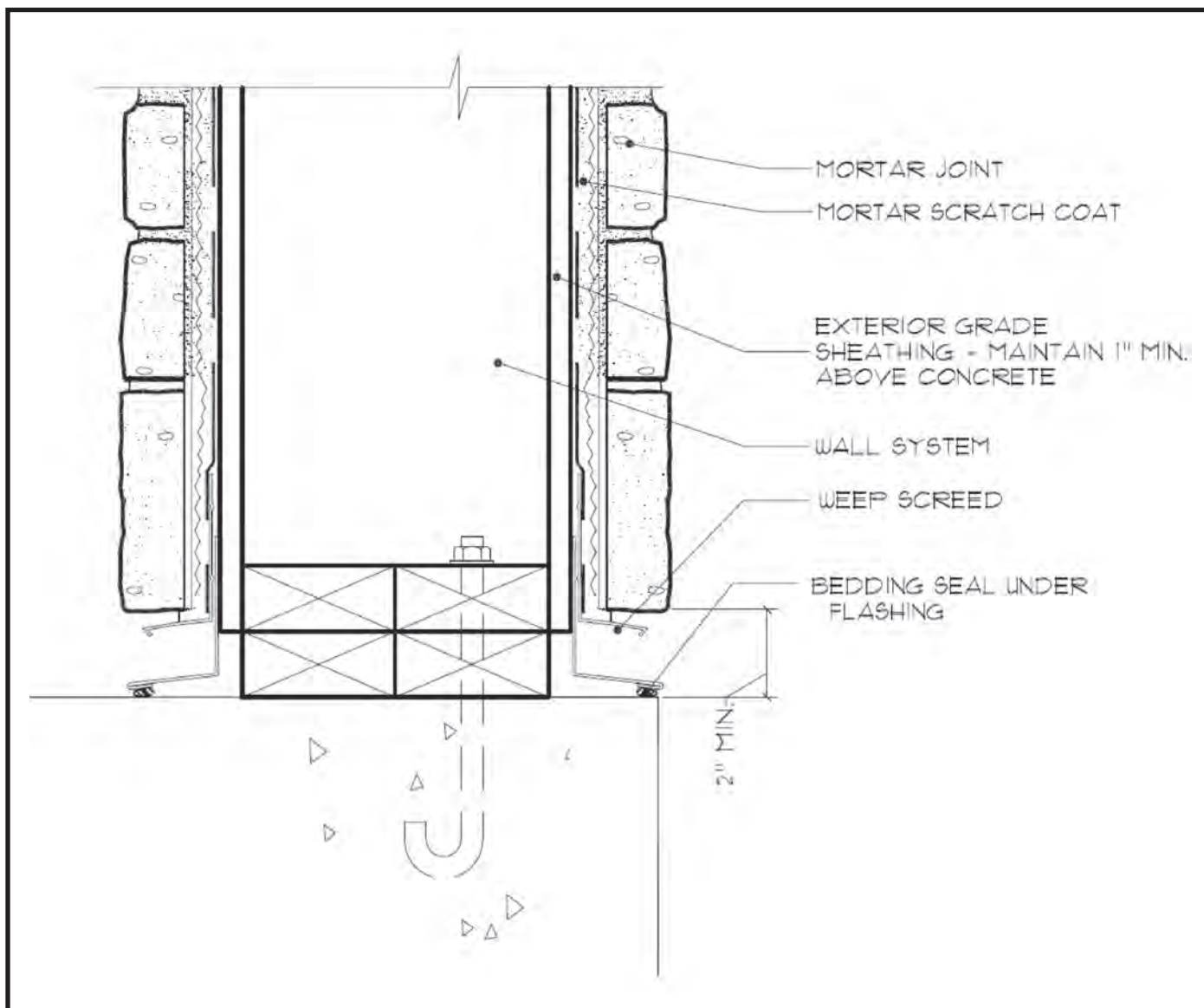
Fig. 25. Column Base
