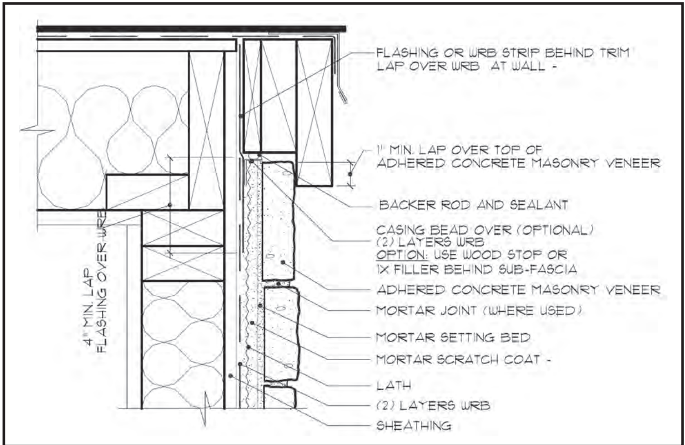
Fig. 14. Rake - Flush
