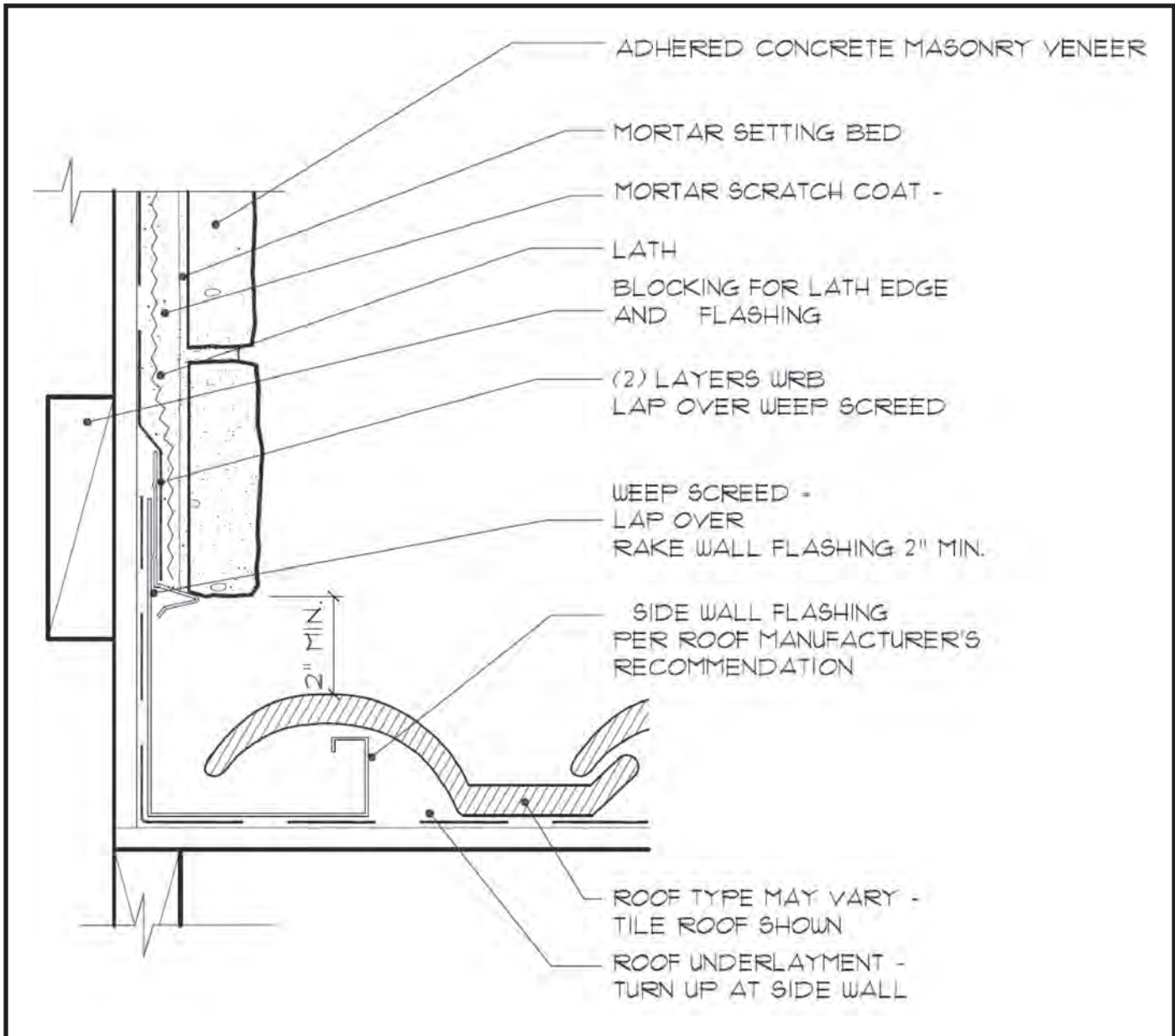
Fig. 17. Side Wall - Tile Roofing
