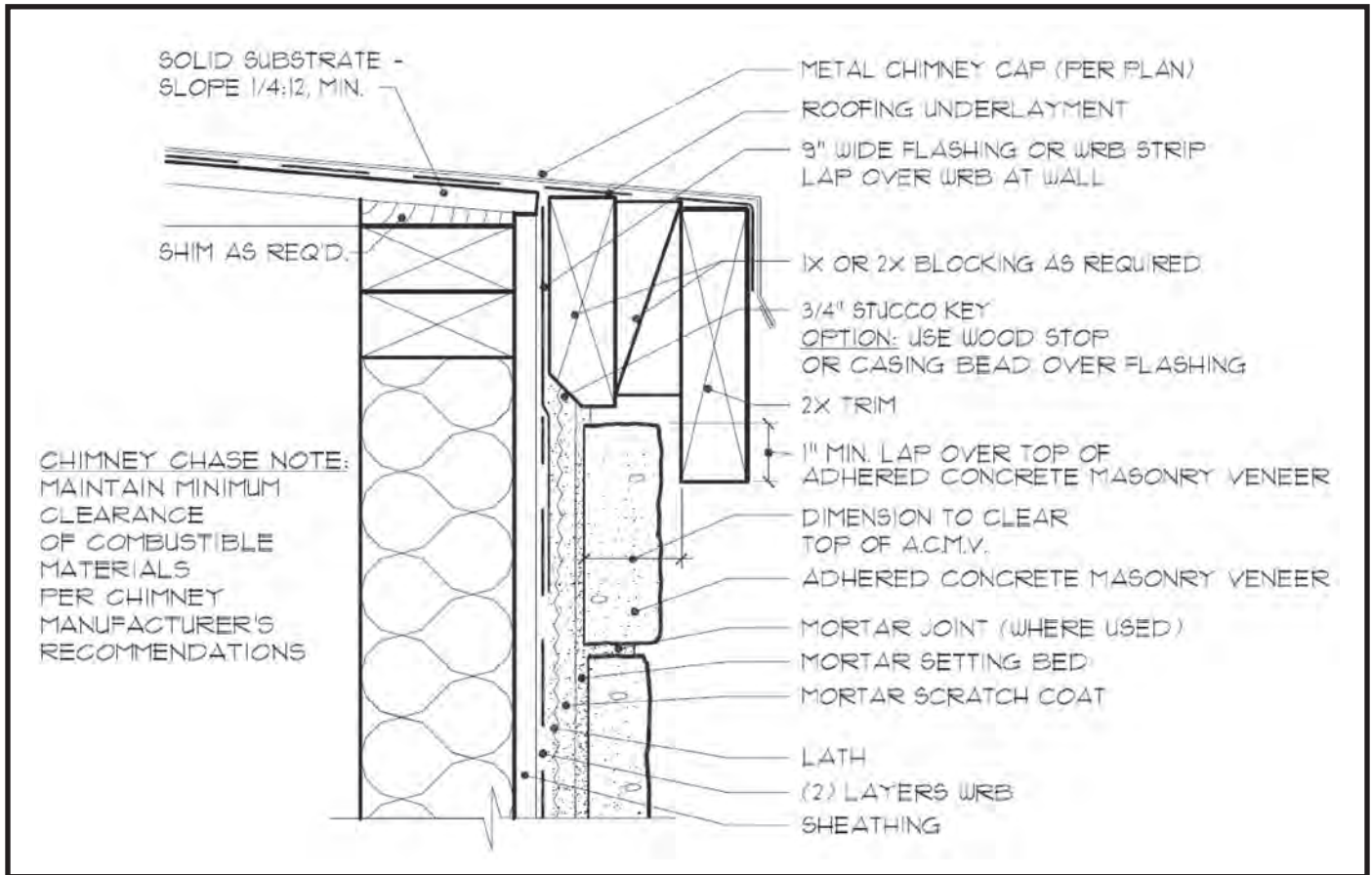
Fig. 24. Chimney Chase
