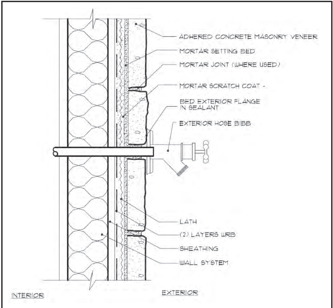
Fig. 28. Pipe Penetration
