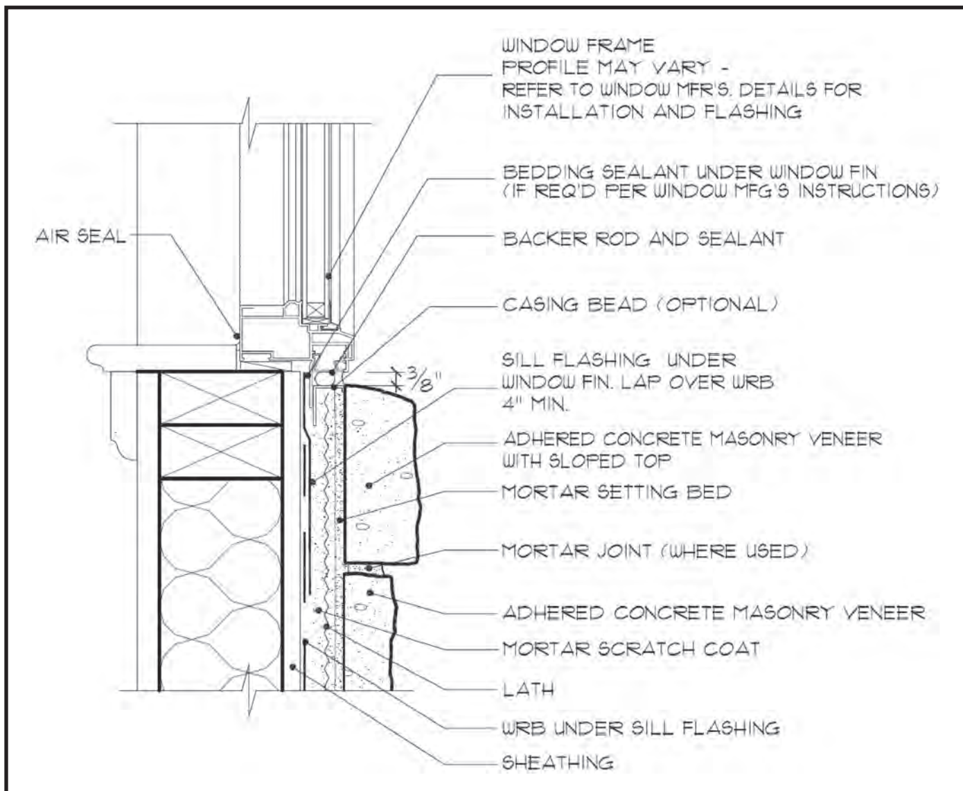
Fig. 19. Window Sill
