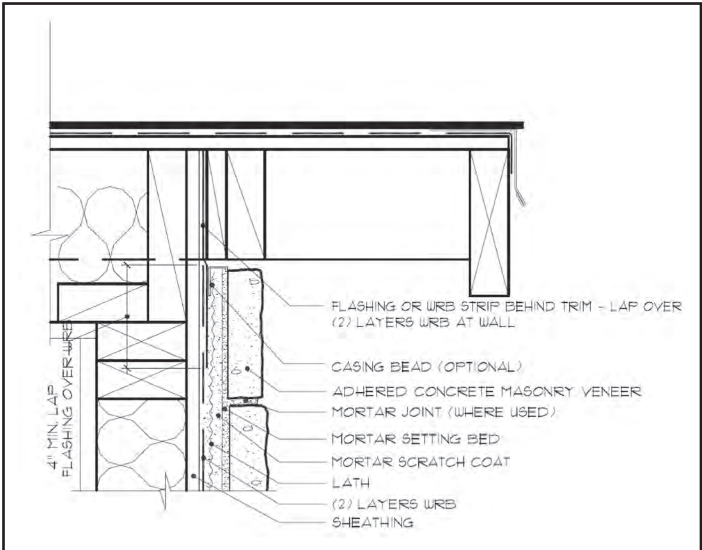
Fig. 13. Rake - Overhang
