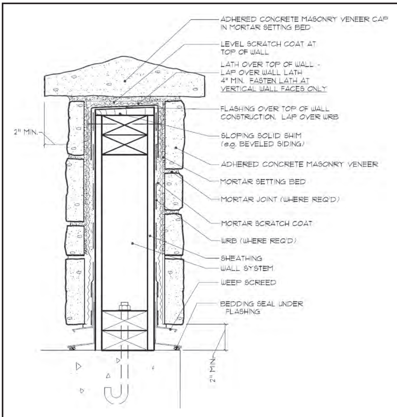
Fig. 31. Wall Cap
